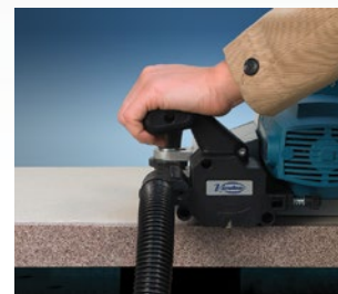
Enrasado de superficies sintéticas (ej. Corian®)
