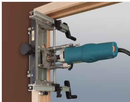
Realización del encaje superior en el marco.
