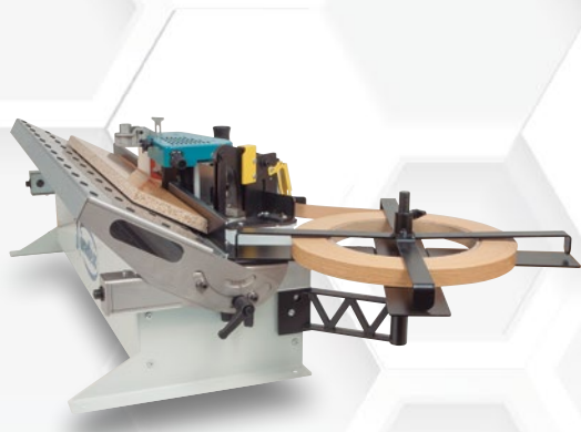
5046703 Perfilador AK97NW + prensos + rodillo (para MEB250, MEB250A)
