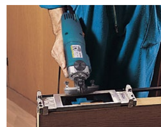
Colocación en la puerta (Mod. A093)
