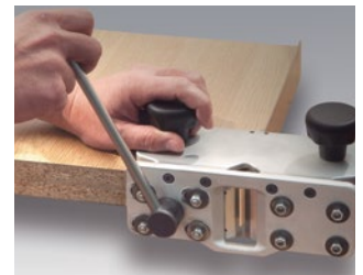
Sistema de corte con dos cuchillas. Equipado con cuchillas afilables de calidad profesional.
