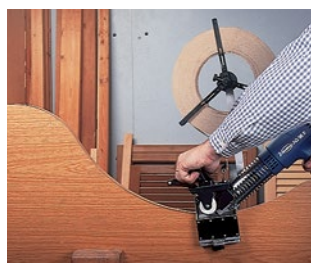
Aplacado de piezas circulares o con formas.
