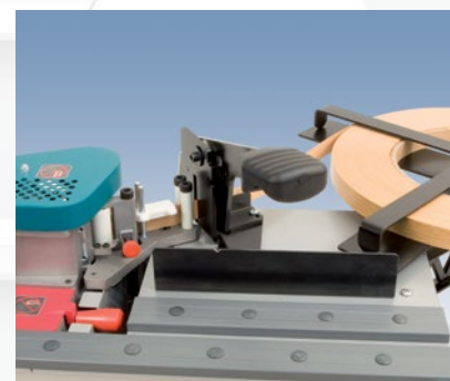
5046266 Cjto cortador + portarrollos RC50T (para MEB250, MEB100)
