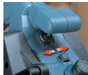
Palanca para la selección del lado de salida de viruta y conexión a un aspirador.
