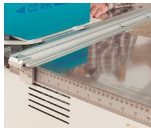
Ajuste fácil de ancho de tira a cortar.
